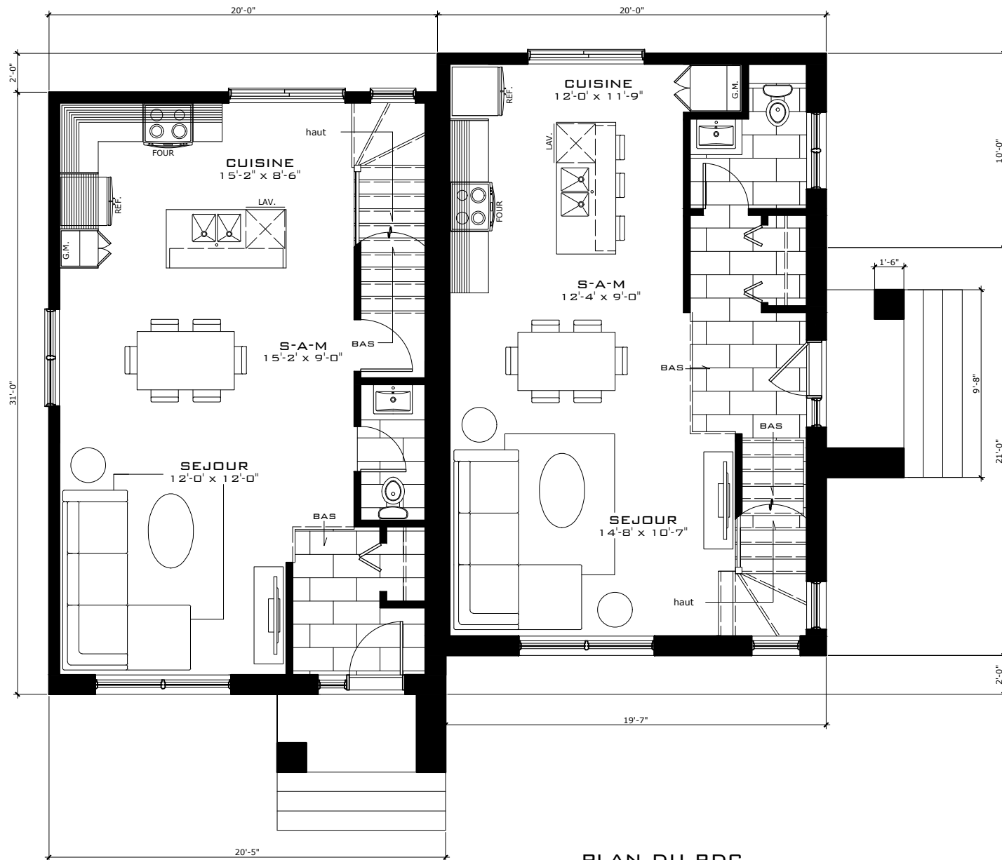
PLAN DU RDC 620 P.I.C.A
