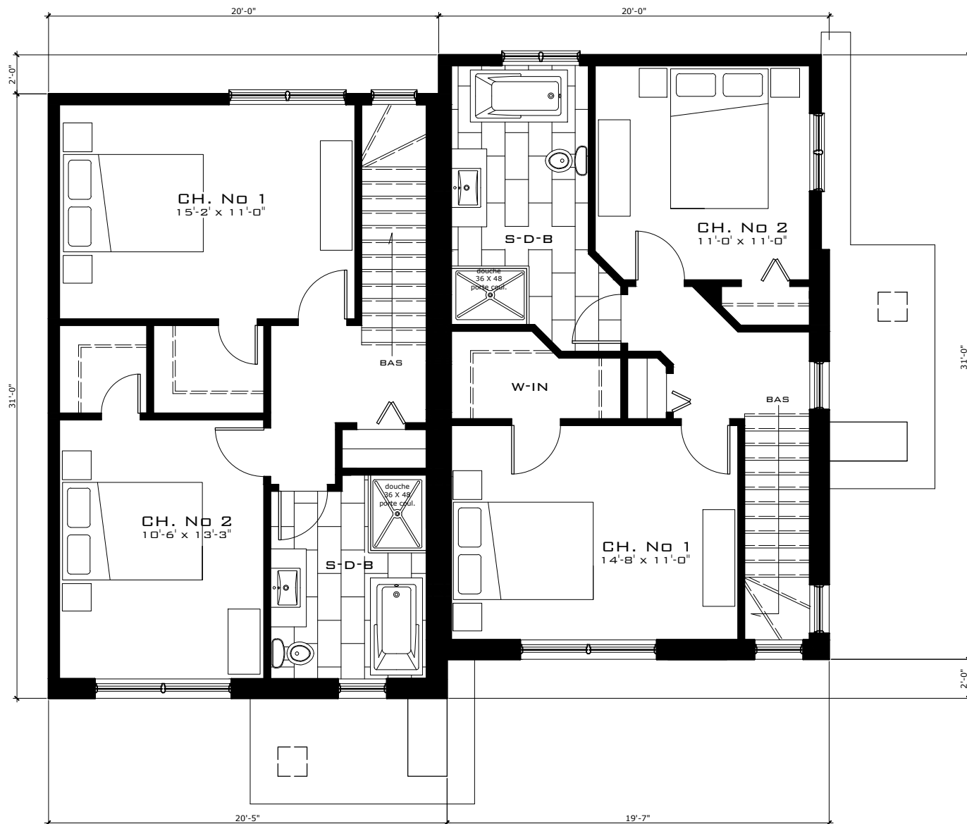
PLAN DE L'ÉTAGE OPTION 2 (MODELE 2 CHAMBRES) 620 PI.CA
